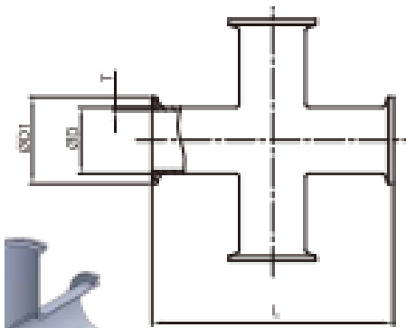
DT-4.1.2-4C CLAMP CROSS (DT-18)
